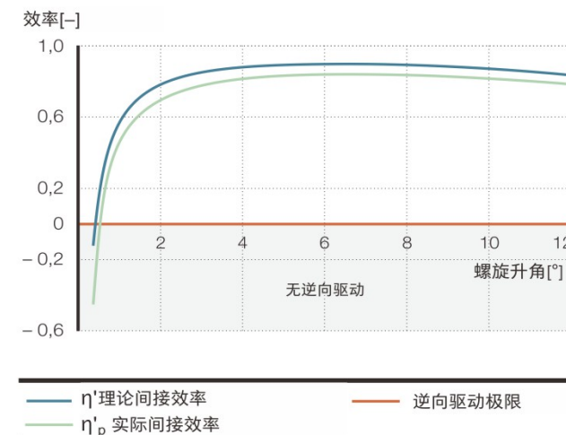
图表3 理论与实际间接效率
