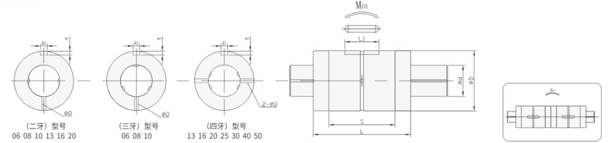
KLT圆筒型
