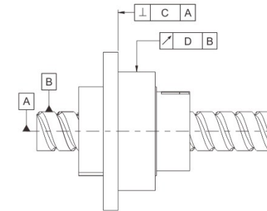
图1.2.3 KFBY系列
