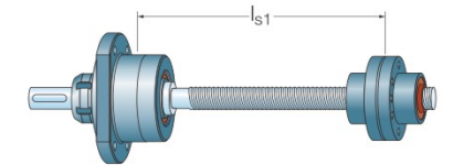
图33 用于刚度计算的带有两个固定支架的配置
