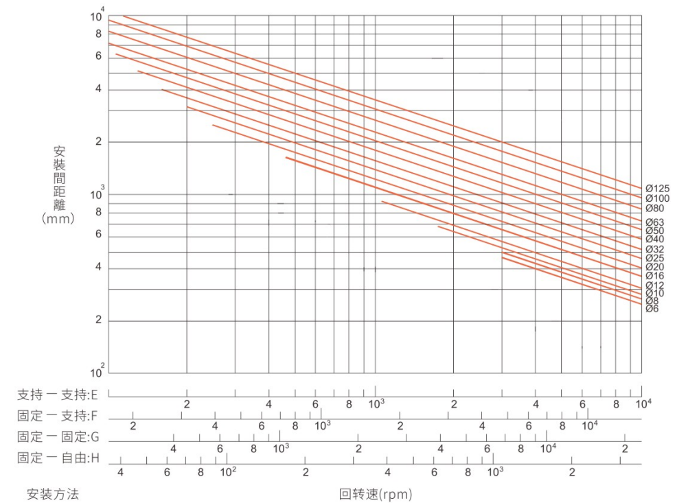
图1.4.17 轴对于危险转速之容许回转速度
