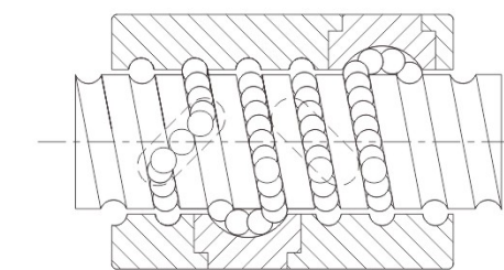
图 1.6.1 U, I, M 型螺帽图
