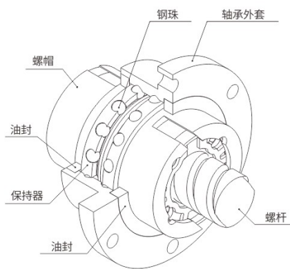
图1.1.4 KFSY 型本体结构
