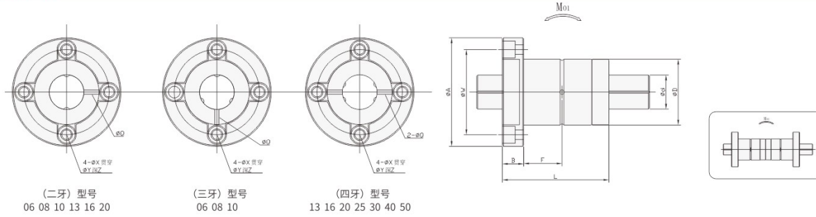
KLF圆法兰型
