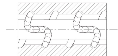
图 1.6.2 K 型螺帽图
