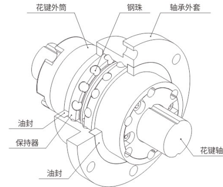
图1.1.5 KLSF 型本体结构
